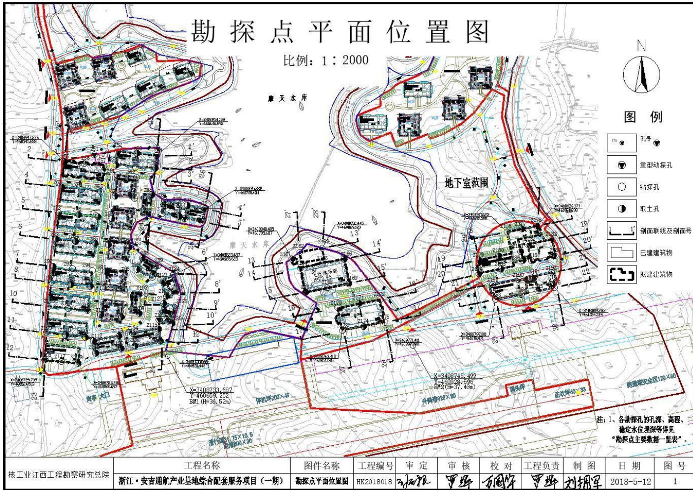
图3-1 工勘地块勘探点平面位置图
