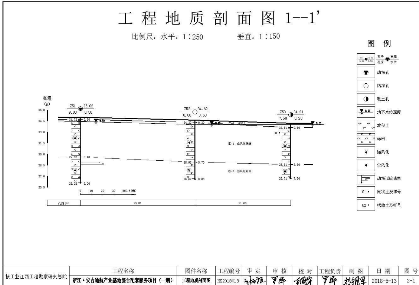
图3-2 工堪地块部分点位工程地质剖面图
